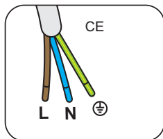
AC power cable (CE) H05RN-F, 3x1.0mm 2
