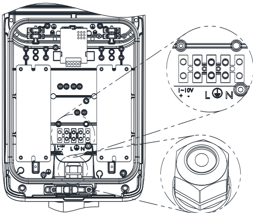
PG M20/M22
