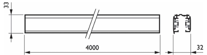
RCS750 5C6 L4000 ALU (XTSC6400-1)
