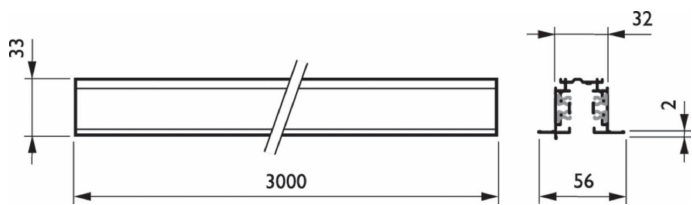
RBS750 5C6 L3000 ALU (XTSCF6300-1)
