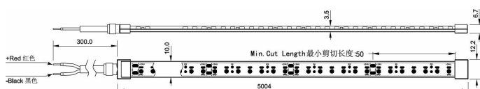
LS170S LED16 927 IP65 L5000 PRO G2
