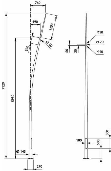
YHB709 CUR 6000 SPK 2xHOLE-M8-80 RAL
