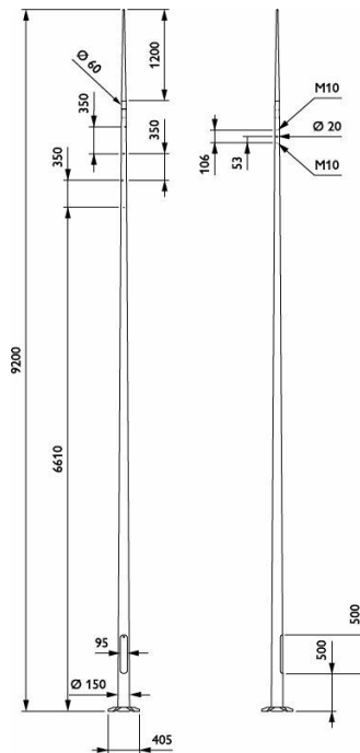
YHB709 CONE 8000 4x2xHOLE-M8-100 RAL
