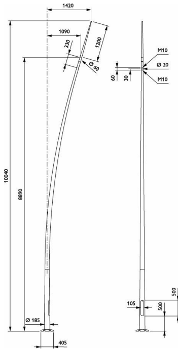
YHB709 CUR 9000 SPK 2xHOLE-M8-80 RAL
