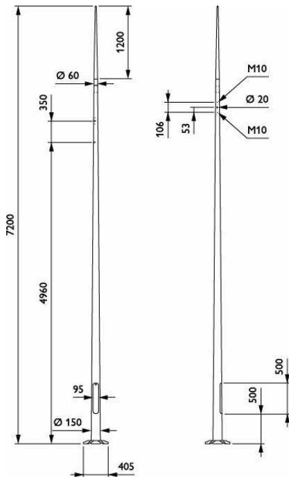
YHB709 CONE 6000 3x2xHOLE-M8-100 RAL
