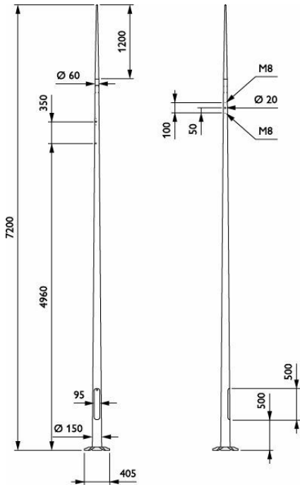
YHB709 CONE 6000 3x2xHOLE-M8-100 RAL
