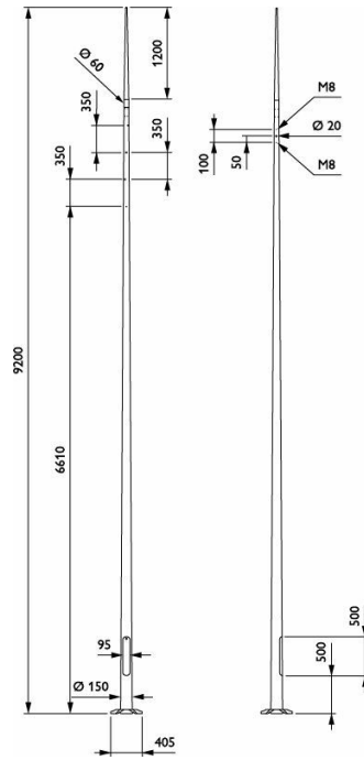
YHB709 CONE 8000 4x2xHOLE-M8-100 RAL
