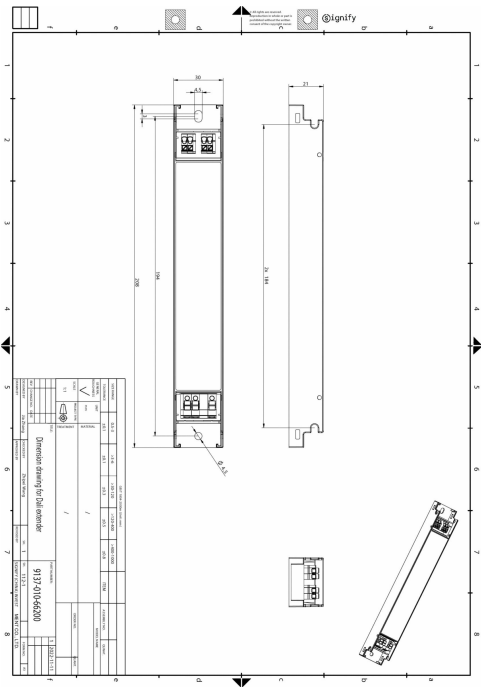
DALI Extender
