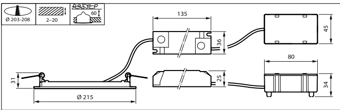
DN145B LED105/830_840 PSU WH
