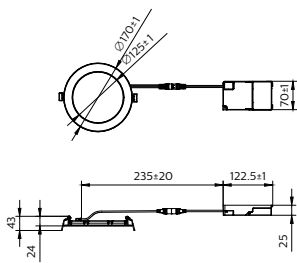
DN145B LED105/830_840 PSU WH
