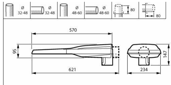
UniStreet gen2 Mini - dimensional drawing
