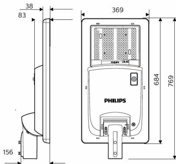
BRP710 LED20 WW 28PO PDIM50 BLE Solar
