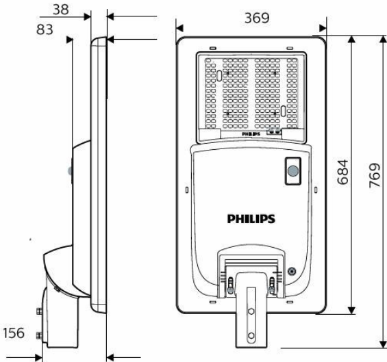
Dimensions
