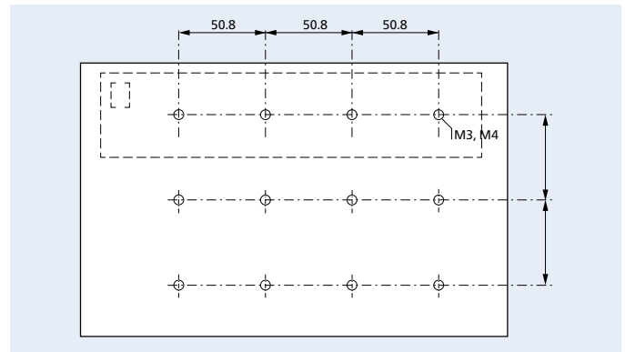
Mounting hole pattern for FastFlex 2x8 DA, DHE
