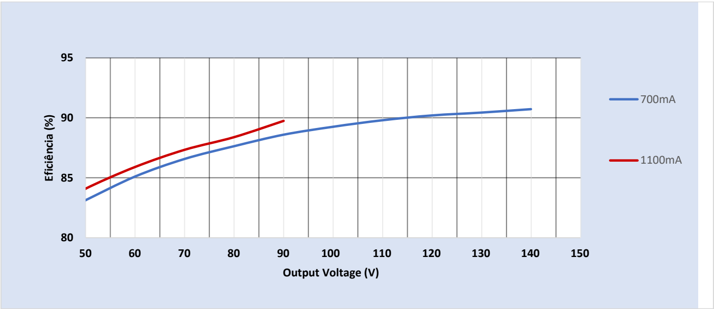
Eficiência Vs. Tensão de saída (Tensão de entrada em 277Vac)
