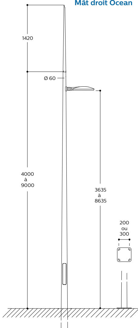
Mât droit Ocean
