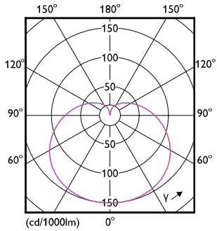
Light Distribution Diagram - LEDBulb 9W B22 DS FR DIM 1PF/6 AU
