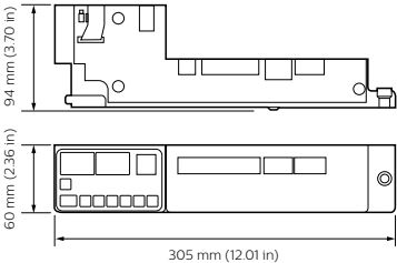
DCM-DyNet
