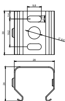
吸顶和吊绳安装支架SM570
