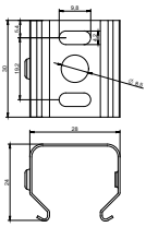
吸頂和吊繩安裝支架SM570
