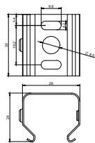
吸頂和吊繩安裝支架SM570
