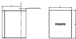
SP570P End Cap W6 L60
