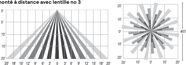
IMRI3 Luminaire ou contrôleur monté à distance avec lentille no 3
