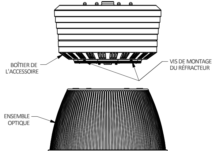
Installation de l'ensemble optique
